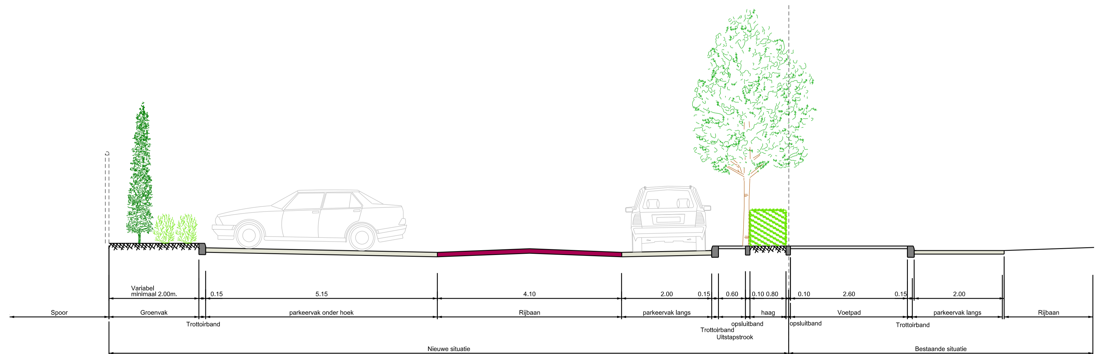
Dwarsprofiel A parkeerterrin Spoorlaan Schaal 1 : 50
